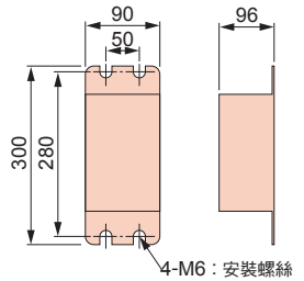
外觀尺寸 mm
