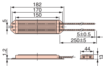
ERF-150WJ 系列
