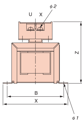
外觀圖 1
