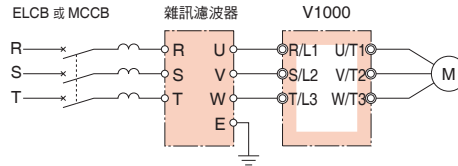
三相輸入時 (LNFD 型、FN 型)
