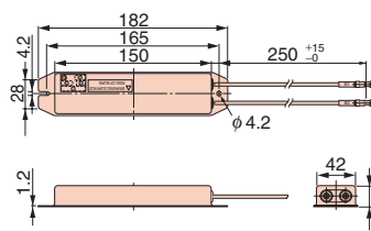
CF120-B579 系列
