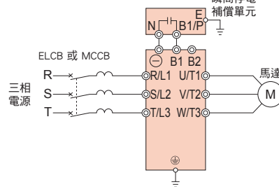
連接圖
