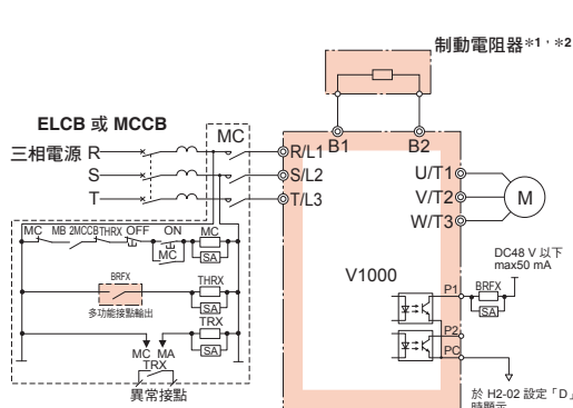
連接圖 A
