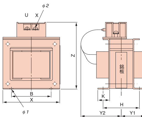
外觀圖 2
