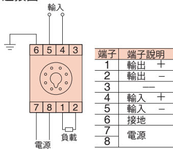
連接圖
