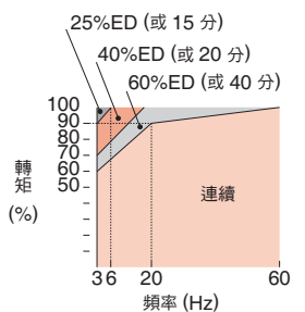
本公司標準馬達之容許負載特性
