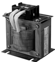
外觀尺寸 mm
