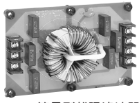
簡易型雜訊濾波器 (無外殼)
