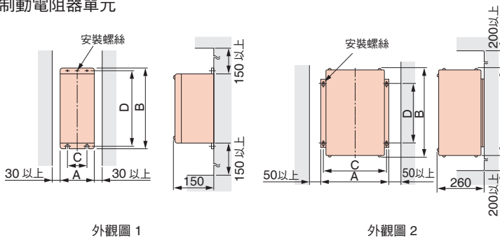
外觀圖 1
