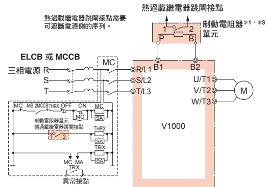
連接圖 B
